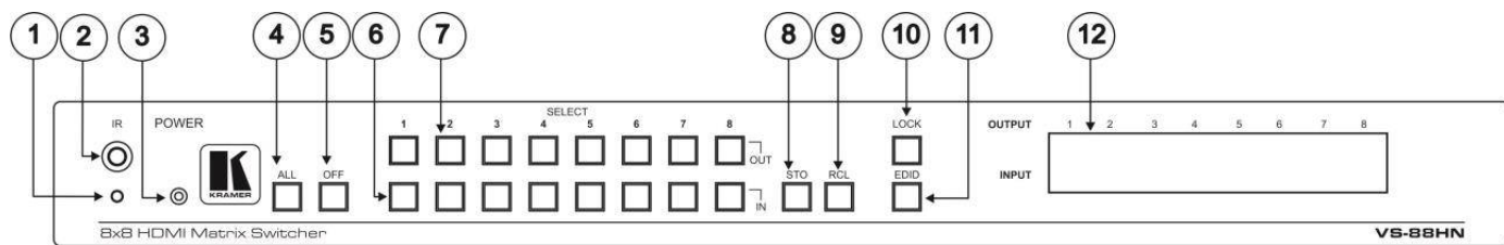
図 1 : VS-88HN 8x8 HDMI マトリックス スイッチャー フロントパネル
