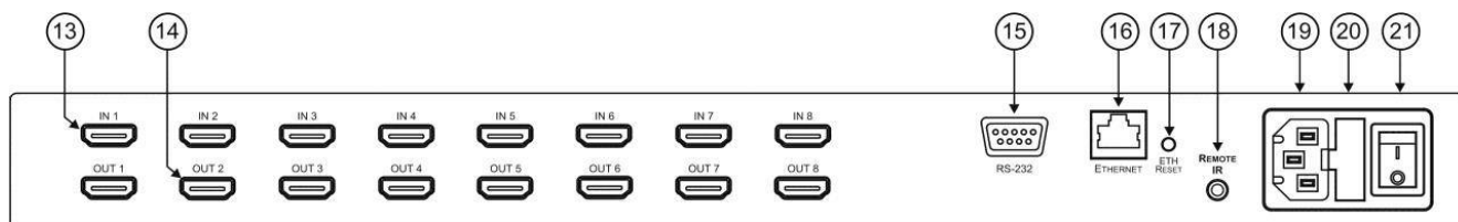
図2: VS-88HN 8x8 HDMI マトリックス スイッチャー リアパネル
