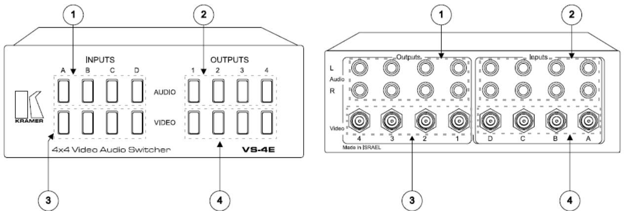
図 1 : VS-4E 4X4 ビデオ オーディオ スイッチャー
