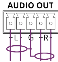
図4：バランスステレオ音声機器への接続
