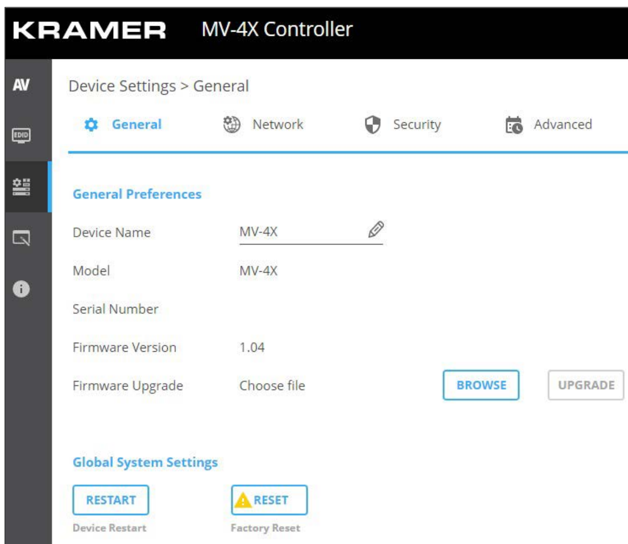
図31 : MV-4X デバイス設定 - General
