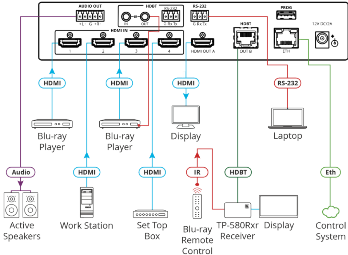
図3 : MV-4Xリアパネルの接続
