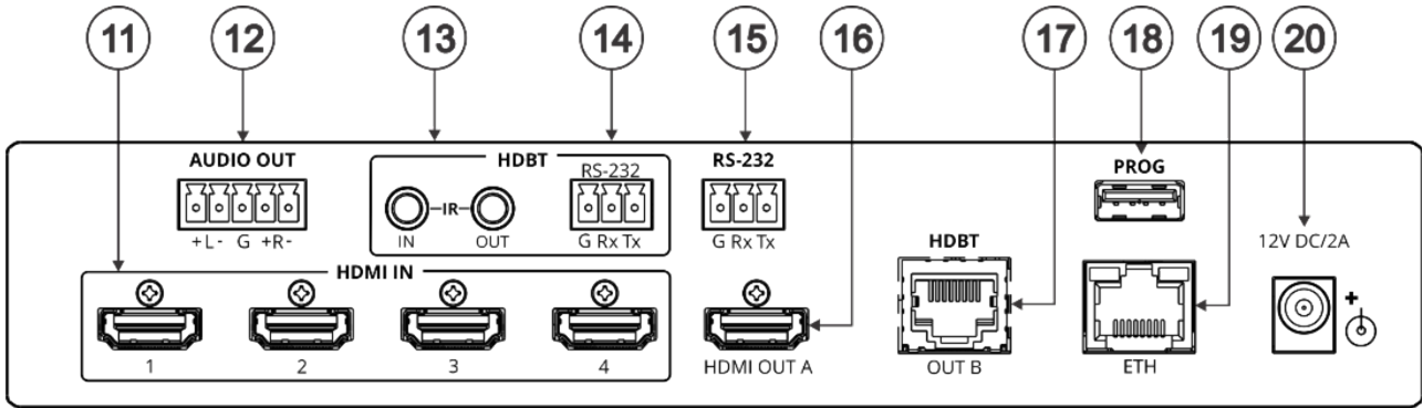
図2 : MV-4X 4ウィンドウマルチビューワ/4x2シームレスマトリックススイッチャー リアパネル
