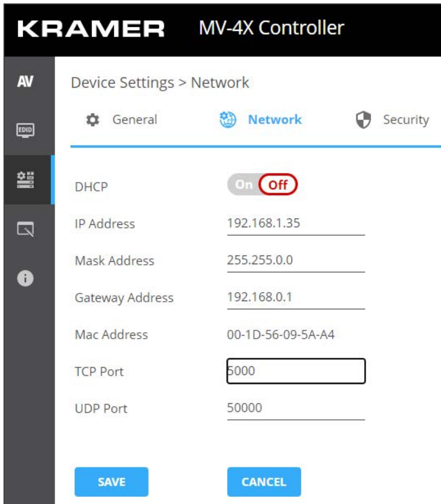
図33：デバイス設定 - ネットワークタブ
