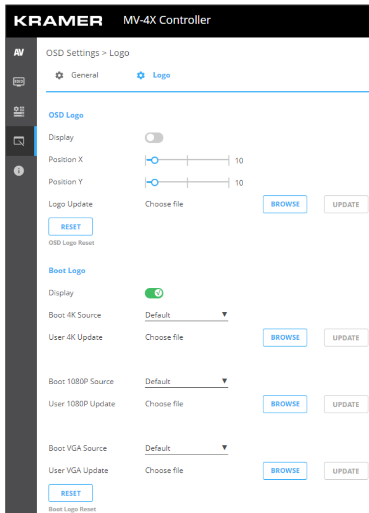
図3：ロゴの設定
