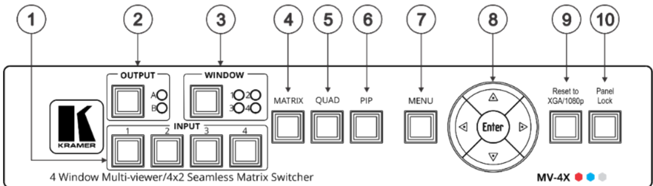
図1：MV-4X 4ウィンドウマルチビューワ/4x2シームレスマトリックススイッチャー フロントパネル
