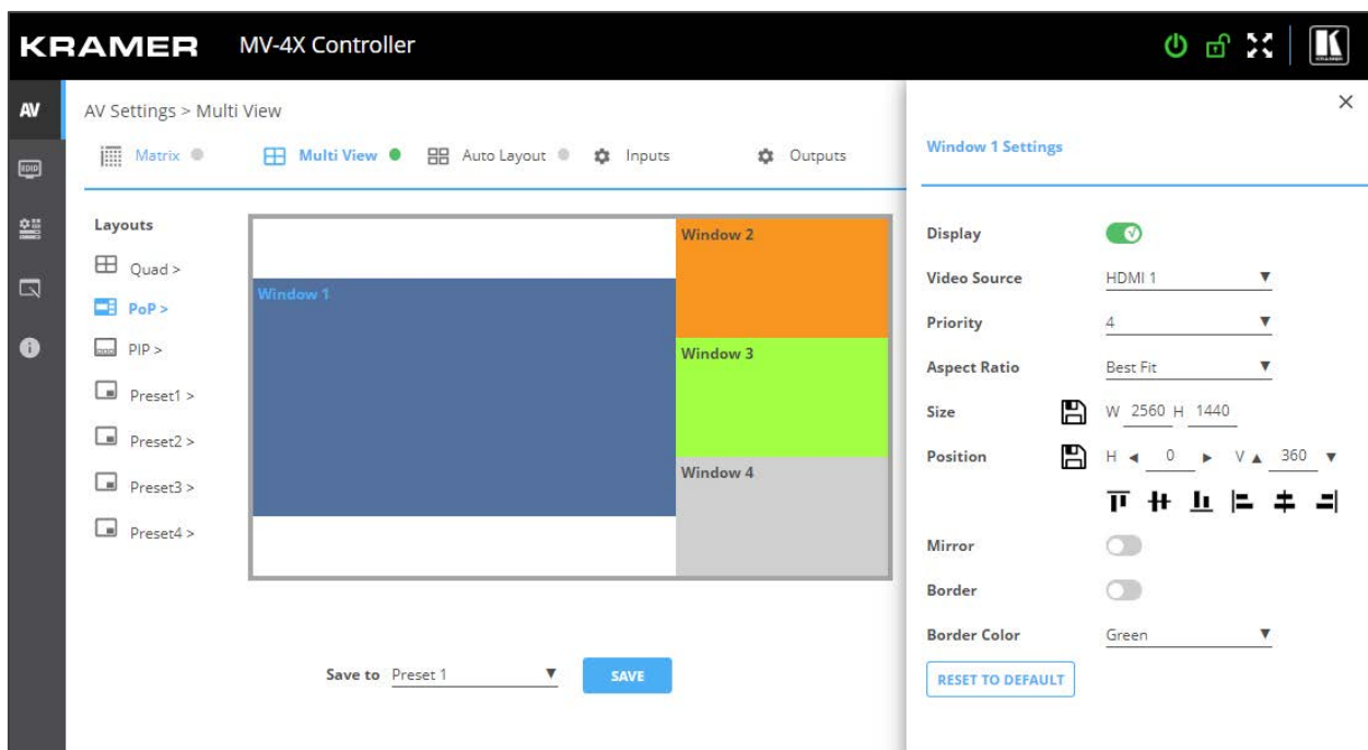
図20：マルチビュータブ - PoPモード
