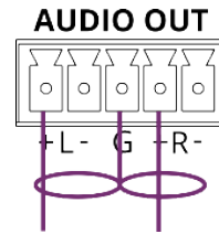
図5：アンバランスステレオ音声機器への接続
