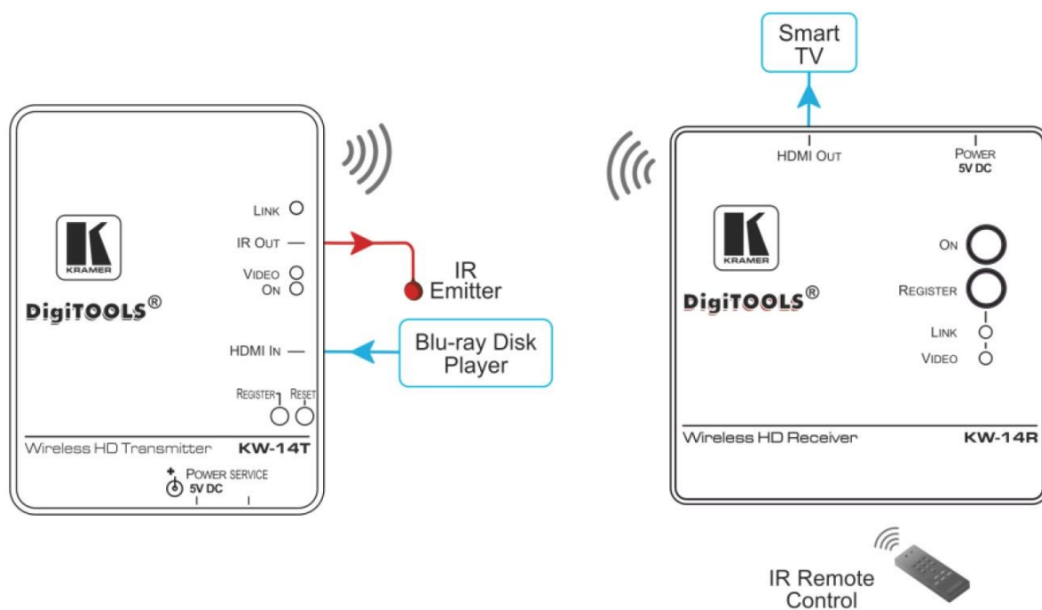
KW-14T、KW-14R 接続例
